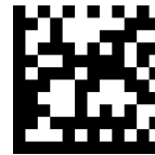
Add TAB
