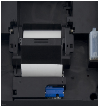
Der Drucker der ECR-1810 ist leicht zu bedienen. Über den SD-Kartenslot stehen das elektronische Journal und Programmiersowie Umsatzdaten zur Verfügung.
